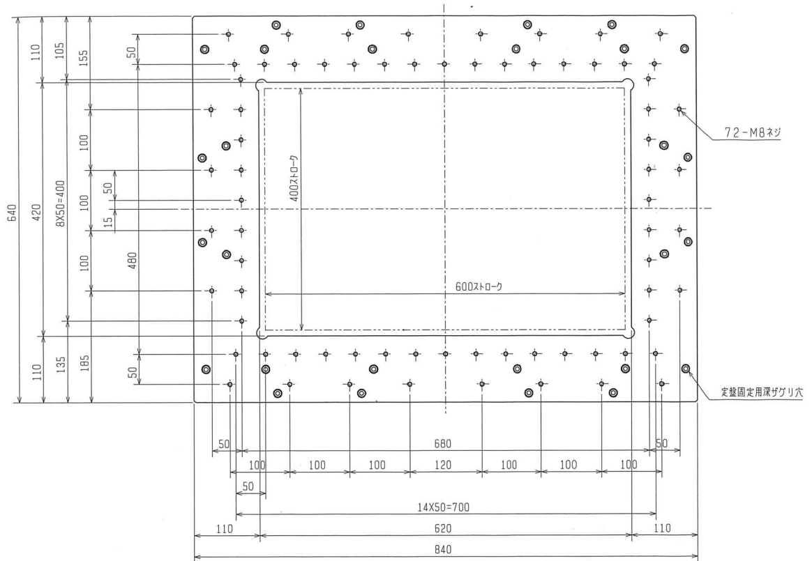
図 1.5.3 MP2400 テーブル定盤（一体ロノ字タイプ）寸法図
