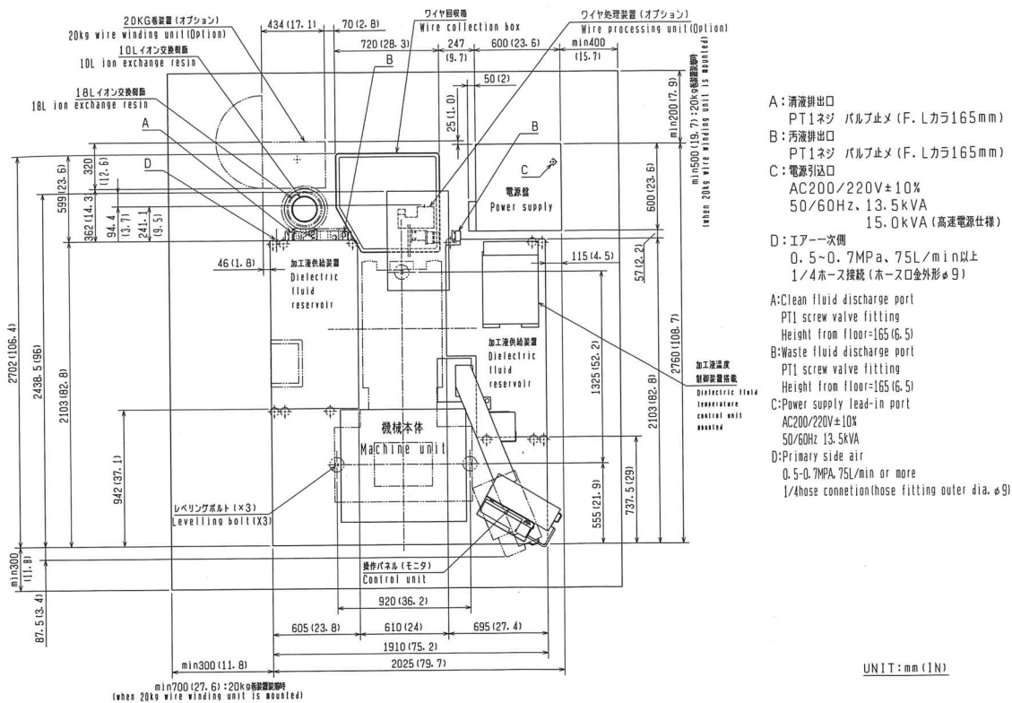
図 1.4.5 MP1200 配置図
