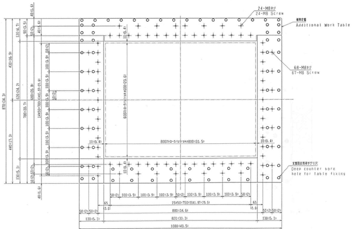
図 1.5.4 MP4800 テーブル定盤（分割ロノ字タイプ）寸法図
