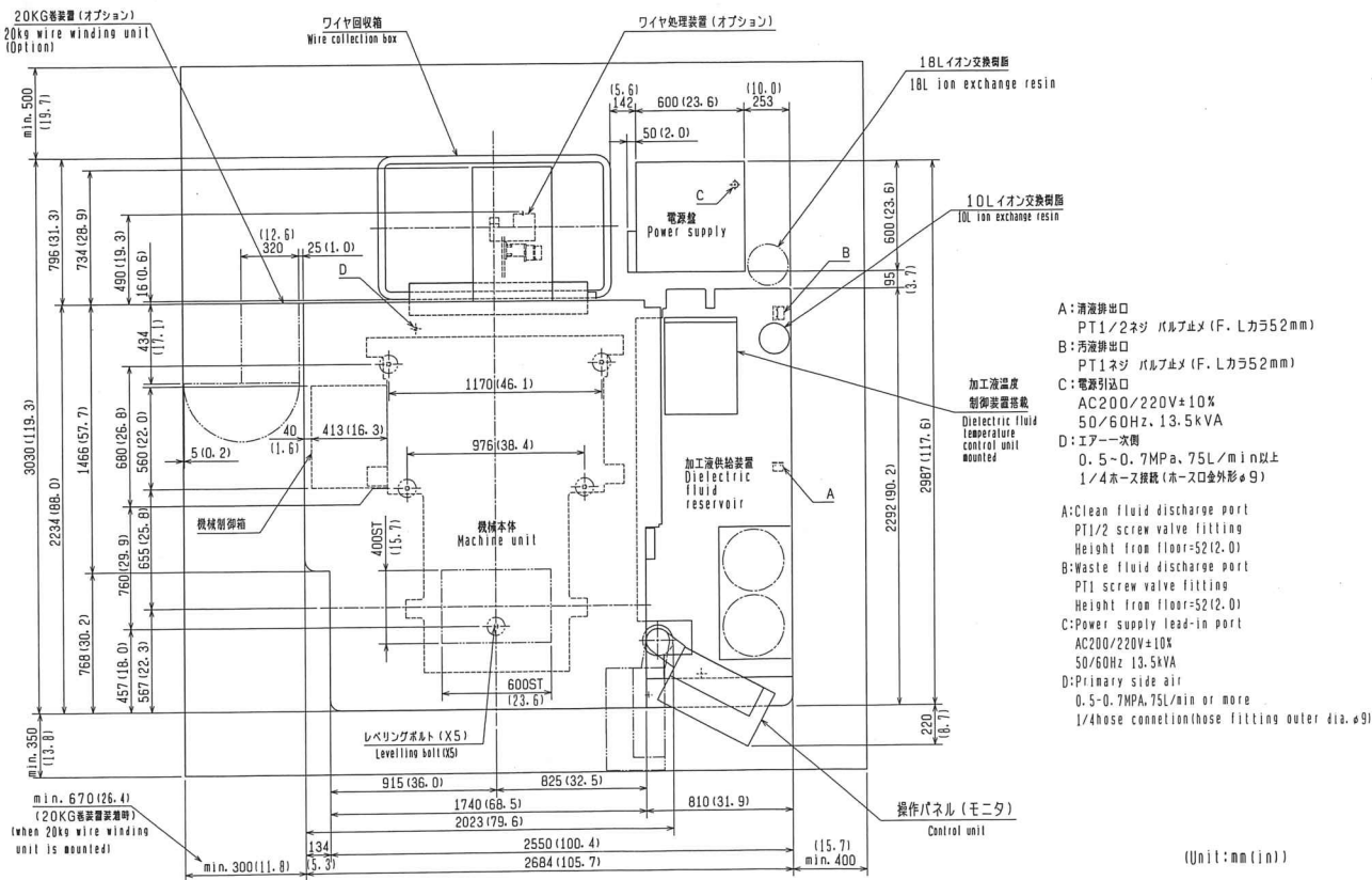
図 1.4.6 MP2400 配置図
