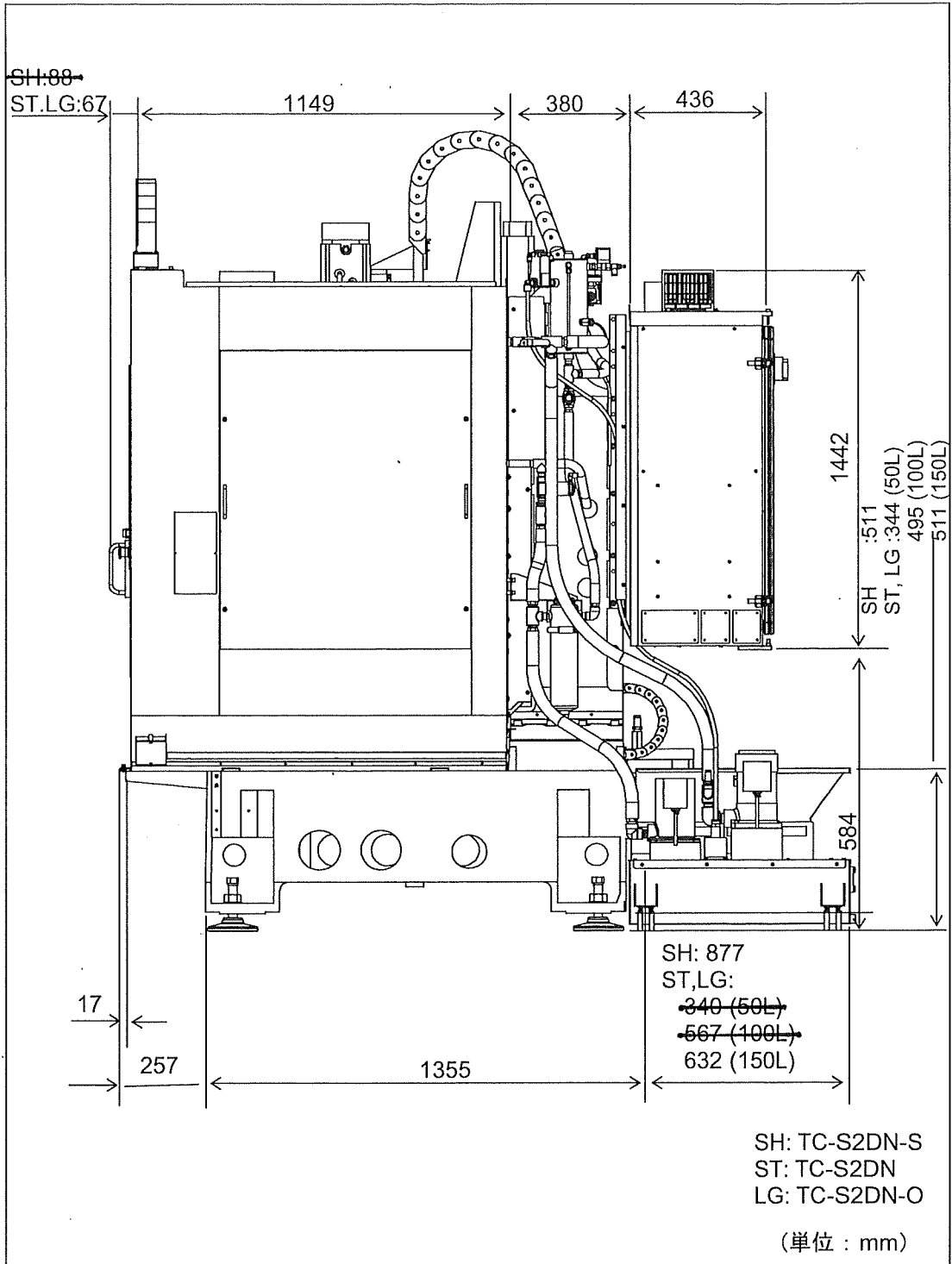
図 2-3 TC-S2DN 外観寸法図 (右側面)
