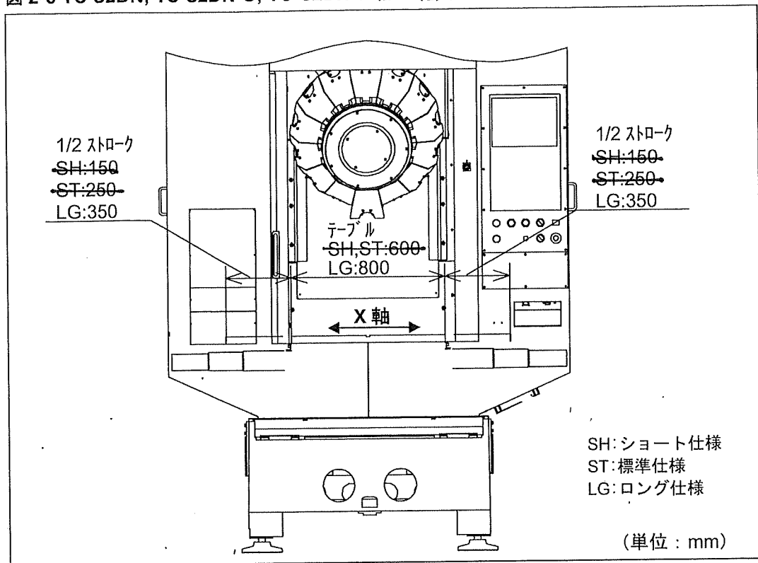
図 2-6 TC-S2DN, TC-S2DN-O, TC-S2DN-S 加工範囲
